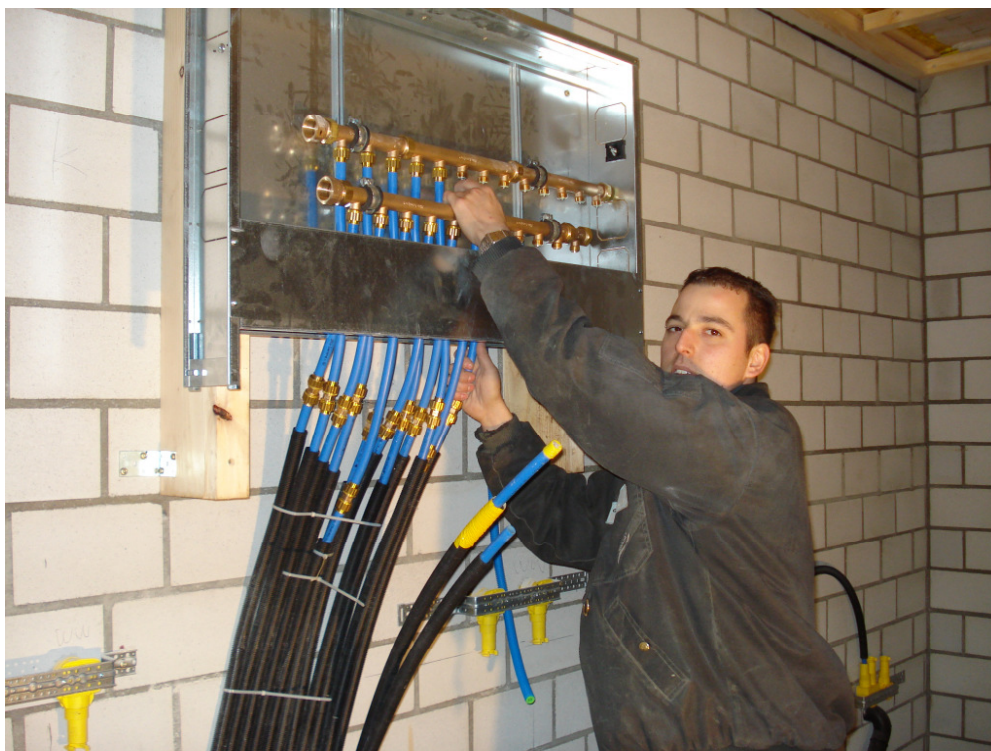
Sanipex-Verteilerkasten
